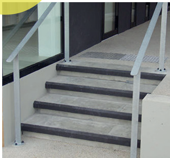
Varningsplattorna placeras innan trappor ca 50 cm från första trappstegets kant.
